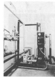
ボイラー
