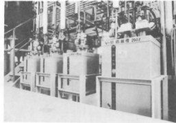
還元剤槽 / 過マンガン酸カリ槽 / 次亜塩素酸ソーダ槽 / 硫酸槽
