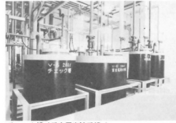
チェック槽 / 重金属廃液受槽 / 水銀廃液受槽 / シアン廃液受槽
